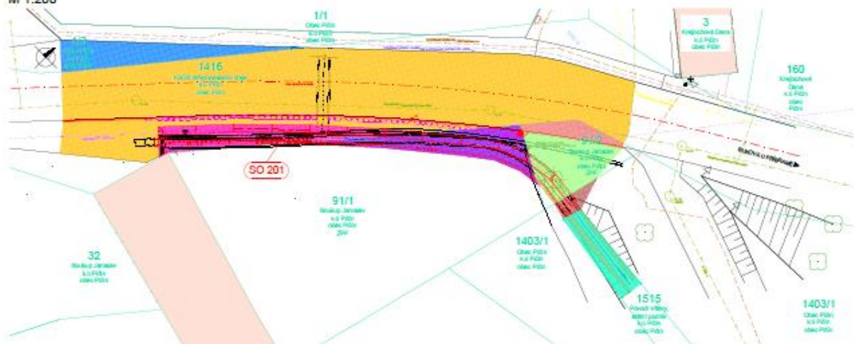
KATASTRÁLNÍ SITUAČNÍ VÝKRES M 1:200
